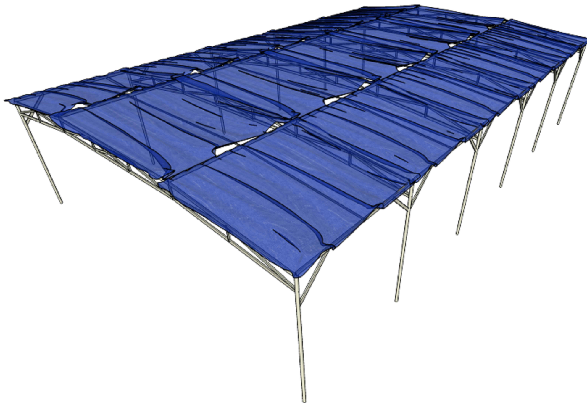
PERSPECTIVA AÉREA COM COBERTURA SEM ESCALA
